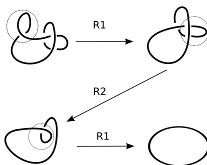
Figura 2: Un esempio: il diagramma rappresenta il nodo banale. Posso infatti "scioglierlo" con una sequenza di 3 mosse di Reidemeister.
