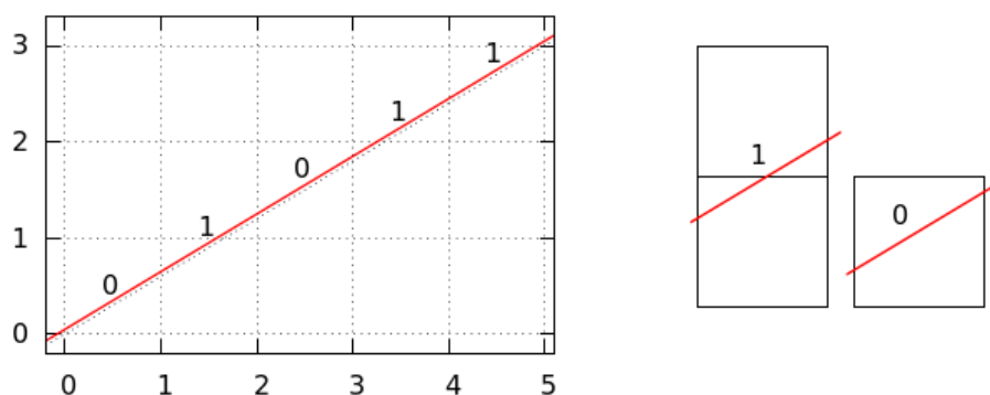
Figura 50: La sequenza di taglio di una retta.
