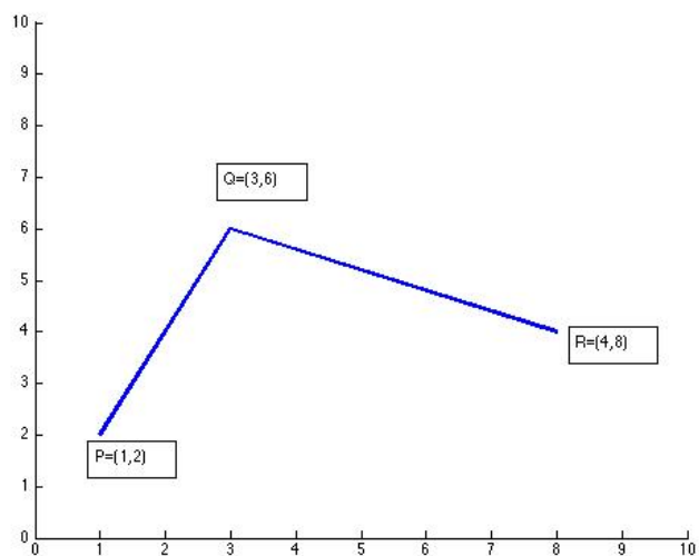
Figura 7: spezzata \overline{PQR}
