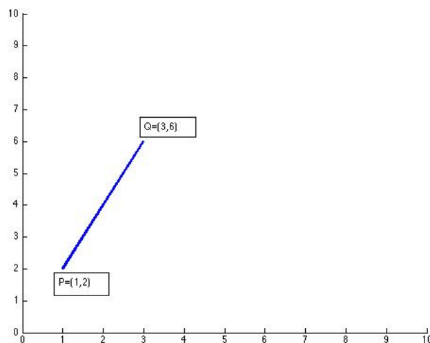
Figura 6: segmento \overline{PQ}
