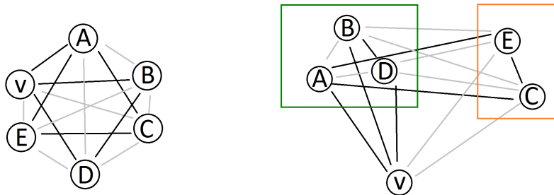
Figura 31: Il processo di isolamento di un vertice.
