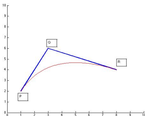
Figura 8: curva che approssima la spezzata PQR
